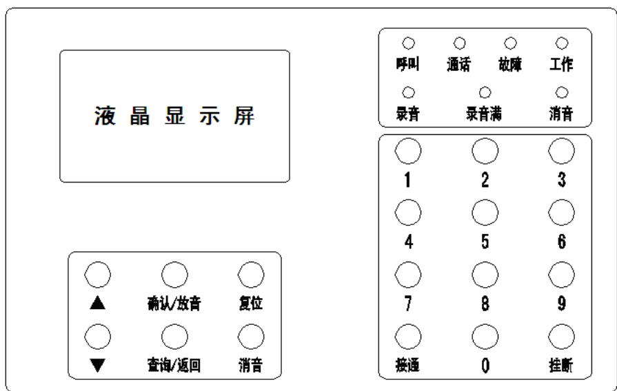
图 4.2 HY5711B 消防电话总机操作显示区示意图
