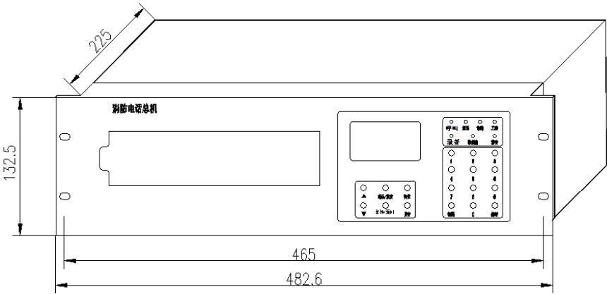
图 4.1 HY5711B 消防电话总机外形示意图
