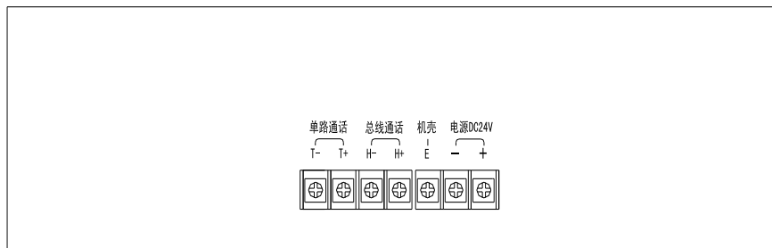
图 3.3 HY5711B 消防电话总机后面板示意图
