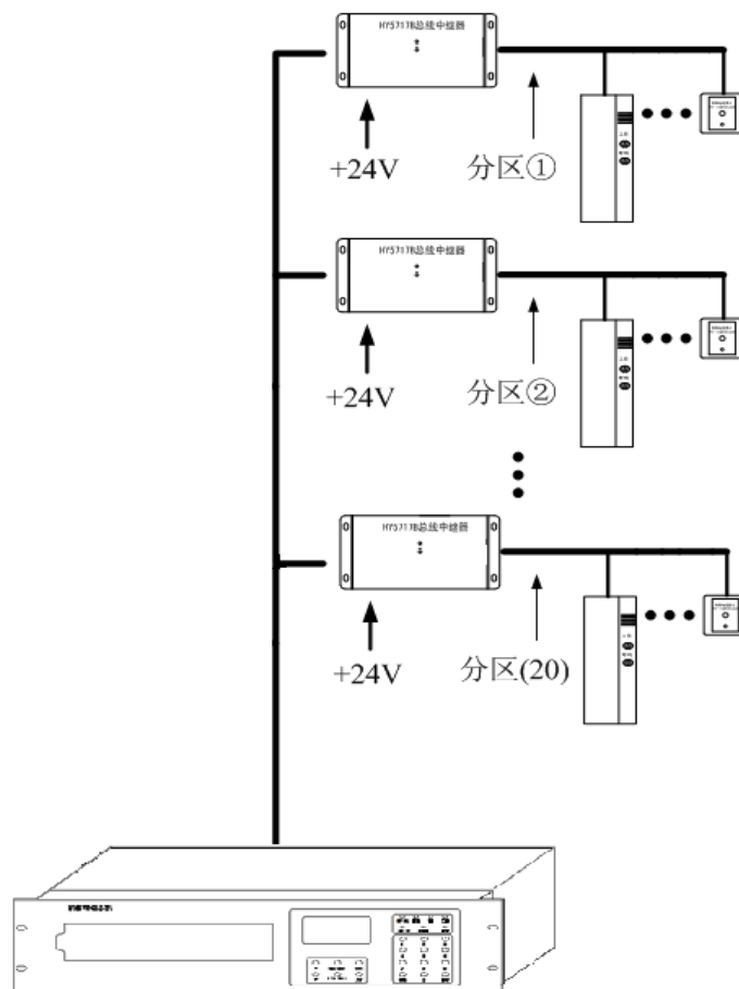
图 3.2 HY5711B 两总线消防电话系统“总线分区”示意图
