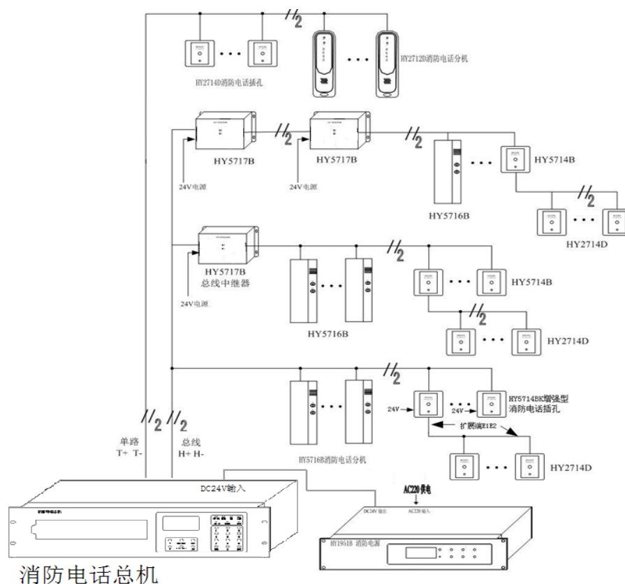
图 3.1 HY5711B 总线消防电话系统构成图
