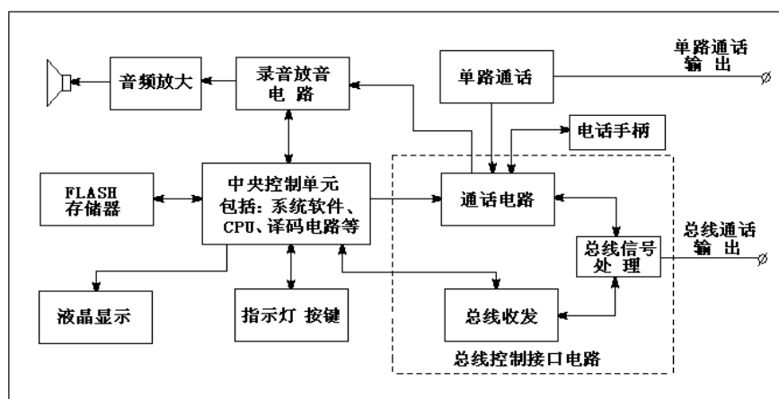
图 3.1 HY5711B 两总线消防电话总机原理结构框图
